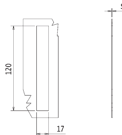
Dima di tranciatura Cutting Template
