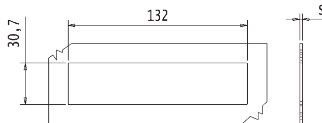
Dima di tranciatura Cutting Template
