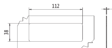
Dima di tranciatura Cutting Template
