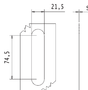
Dima di tranciatura Cutting Template
