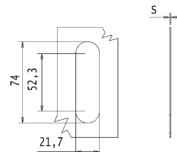
Dima di tranciatura Cutting Template
