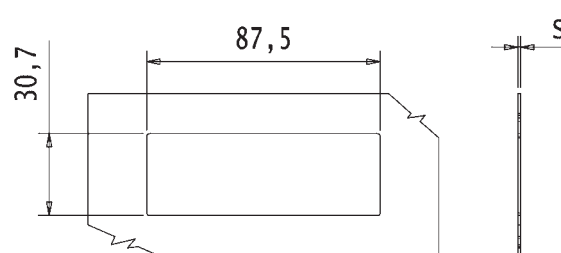
Dima di tranciatura Cutting Template
