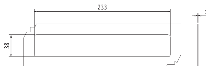
Dima di tranciatura Cutting Template
