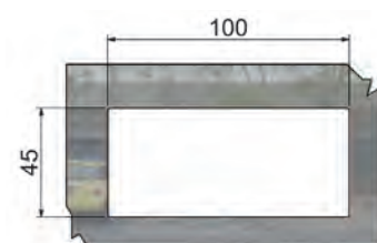
Dima di tranciatura / Cutting Template
