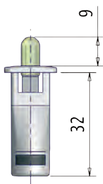
ART. 110 CERNIERA CON MOLLA HINGE WITH SPRING
