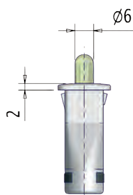
ART. 111 CERNIERA CON PERNO FISSO HINGE WITH FIXED PIN
